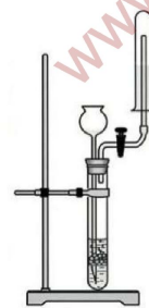
图 1.2-2 简易启普发生器制备氢气, 向下排空气法收集氢气
